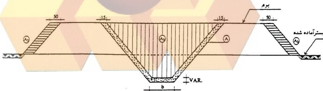
شکل ۳-۳. شمای مقطع خاکبرداری
