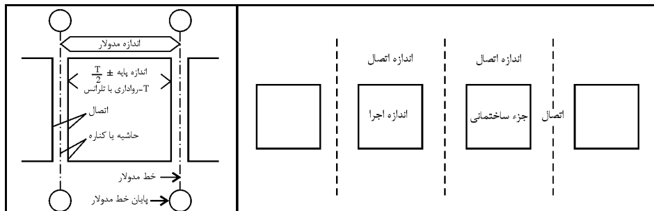
شکل ۱ اندازه مدولار یا هماهنگ‌ساز.
