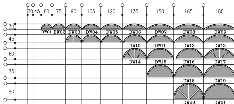
□ ابعاد پنجره های قوسی
