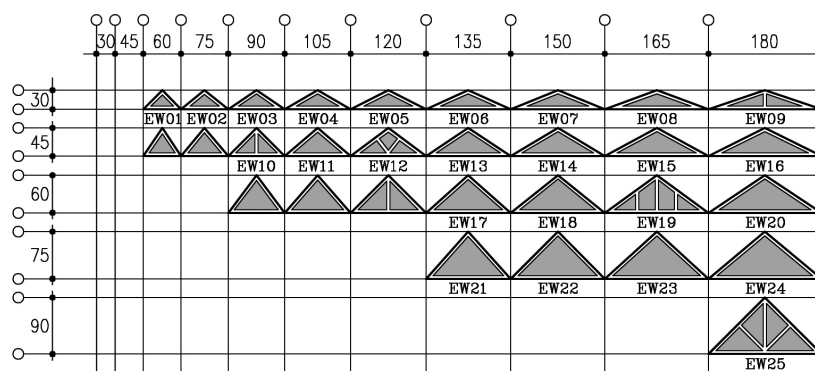
□ ابعاد پنجره های مثلثی
