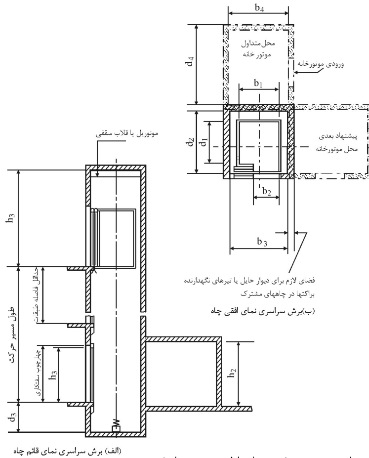
شکل ۳-۳ طرح اولیه معماری آسانسورهای هیدرولیکی مسافری با تردد موردی. (دسته‌های اول، دوم و چهارم)
