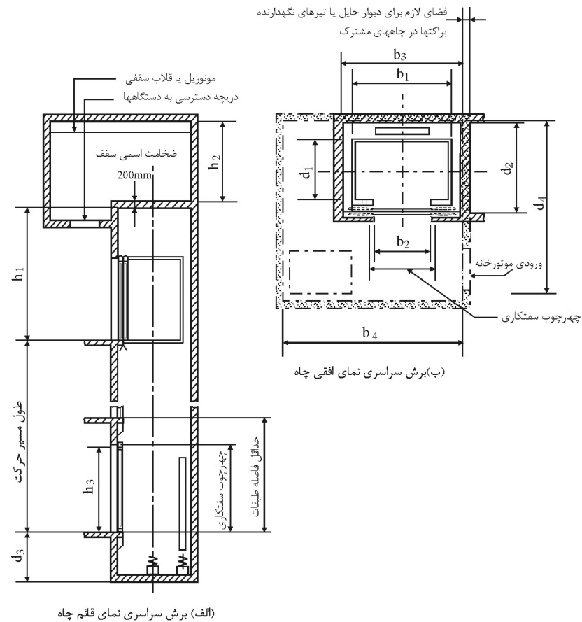
شکل ۵ طرح اولیه معماری آسانسورهای الکتریکی مسافری با تردد زیاد. (دسته سوم با تردد زیاد)
