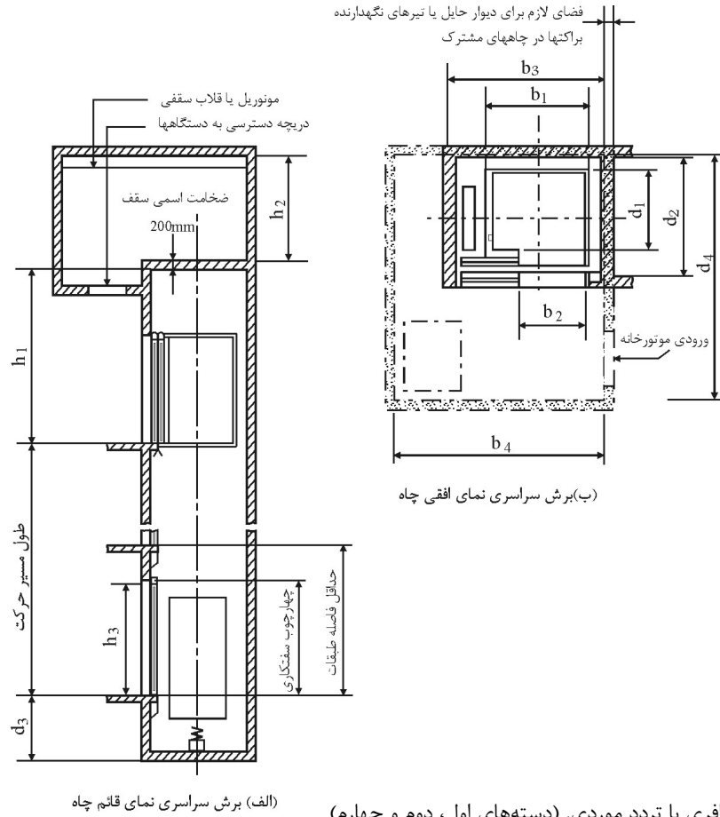
شکل ۳-۲ طرح اولیه معماری آسانسورهای الکتریکی مسافری با تردد موردی. (دسته‌های اول، دوم و چهارم)
