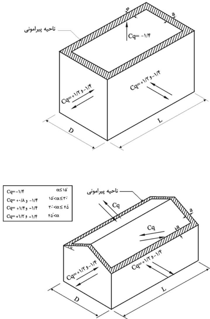
شکل ۶-۶-۳ ضریب شکل C_q برای دیوارها، پوشش بام‌ها و عناصر سازه‌ای نگهدارنده آنها یادداشت: برای بام‌ها بند (۶-۶-۸-۲-ب)، نواحی پیرامونی، نیز باید رعایت شود.
